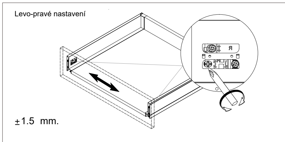
Regulación Izquierda-Derecha / Levo-pravá úprava
