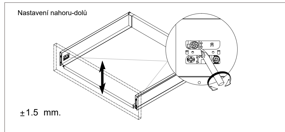
Regulación Arriba-Abajo / Up/down adjustment
